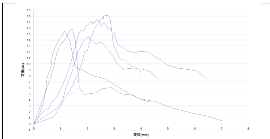
図11:荷重変位曲線
